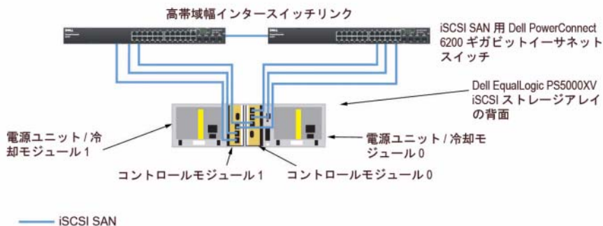
図 8. 推奨ネットワーク構成
